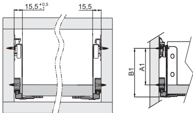
Схема монтажа для метабоксов 350 - 550 мм
