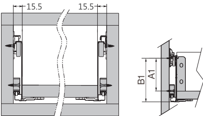
Схема монтажа для метабоксов 250 - 300 мм
