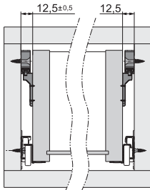
Схема монтажа для роликовых направляющих 350 - 550 мм
