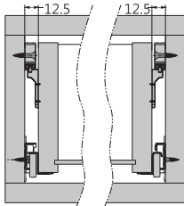
Схема монтажа для роликовых направляющих 250 - 300 мм
